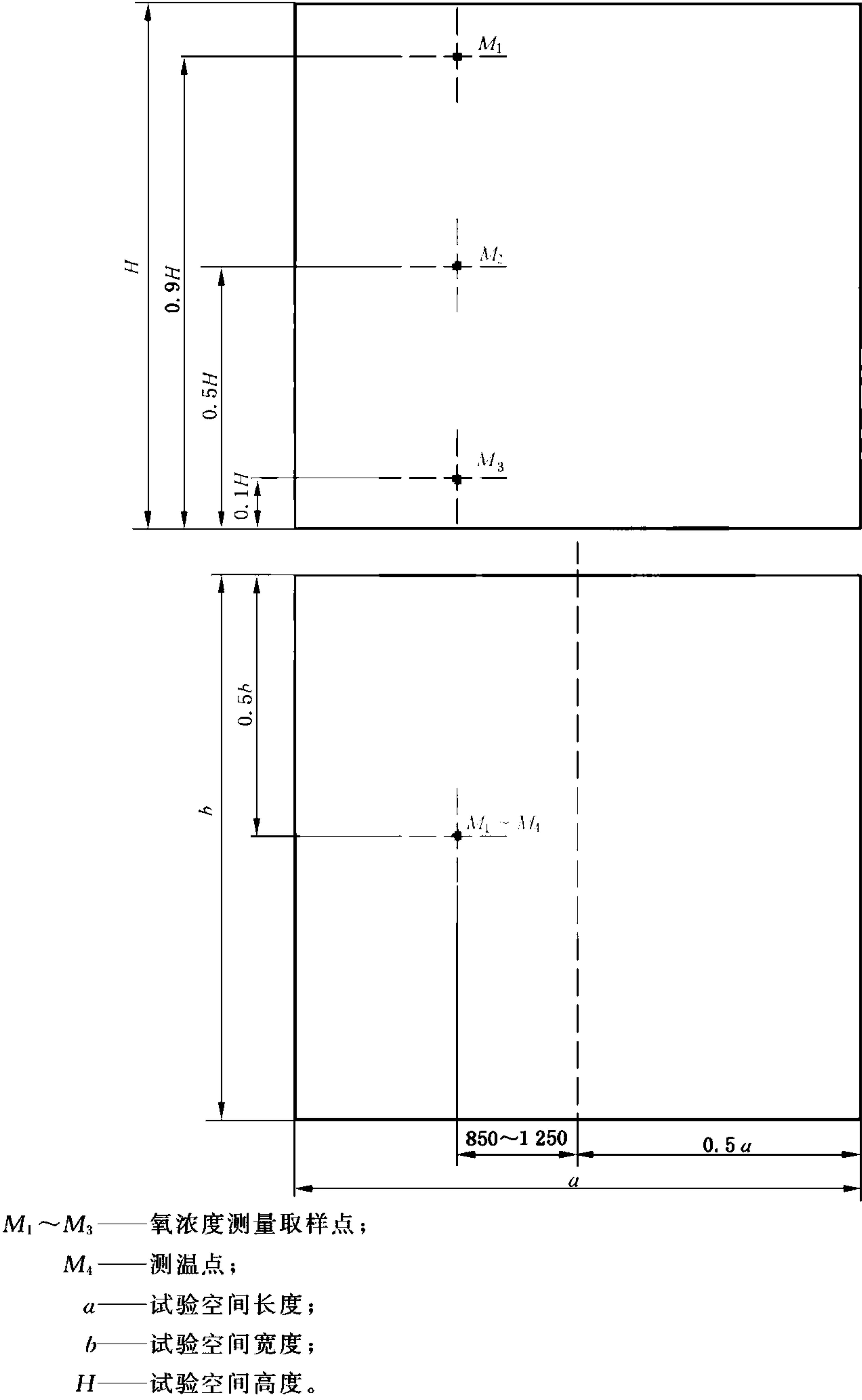
图 6 喷嘴最大安装高度试验测量点布置示意图
